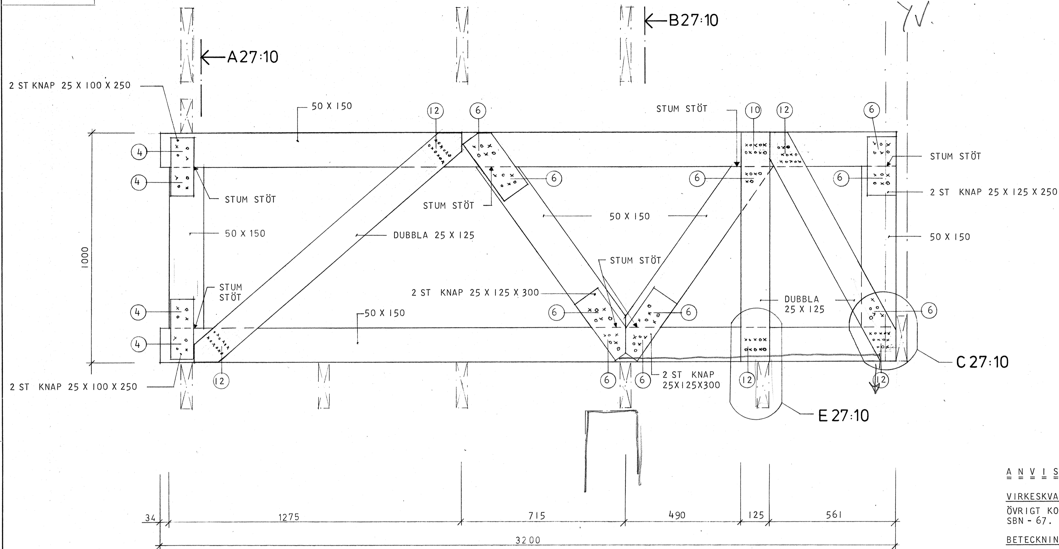
A FACKVERK TYP 4 ANTAL: 1 ST / HUS
